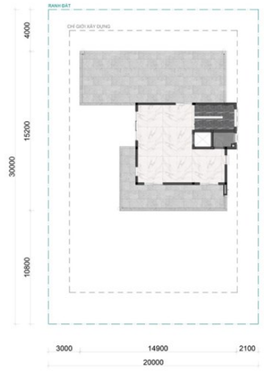
TẦNG 3
